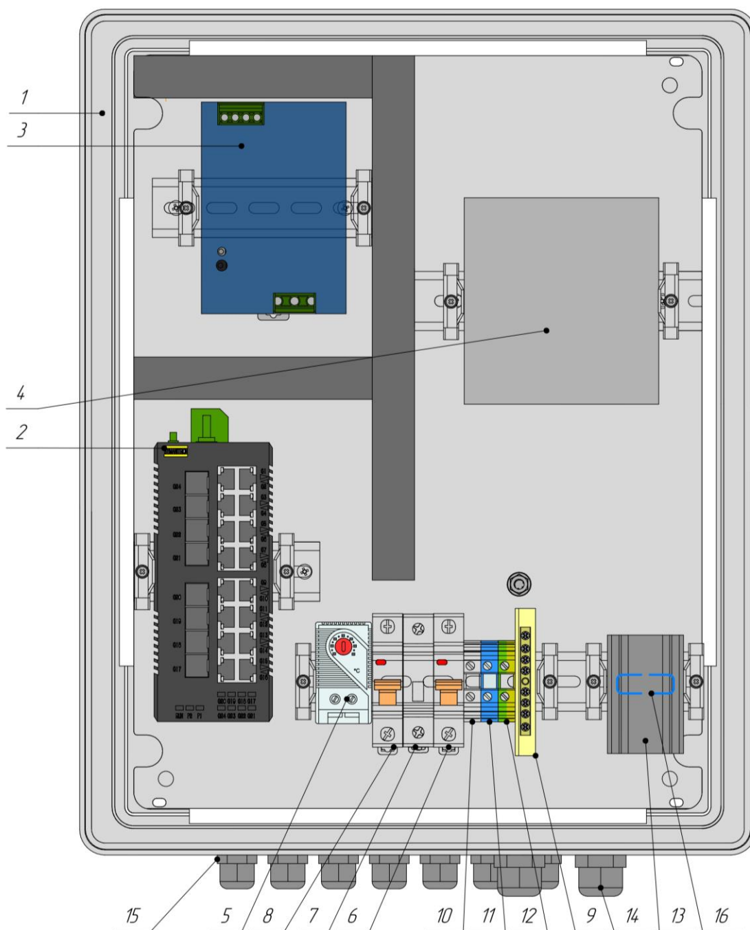
Рисунок 2. Схема расположения оборудования Узла доступа 0168S1-PL
