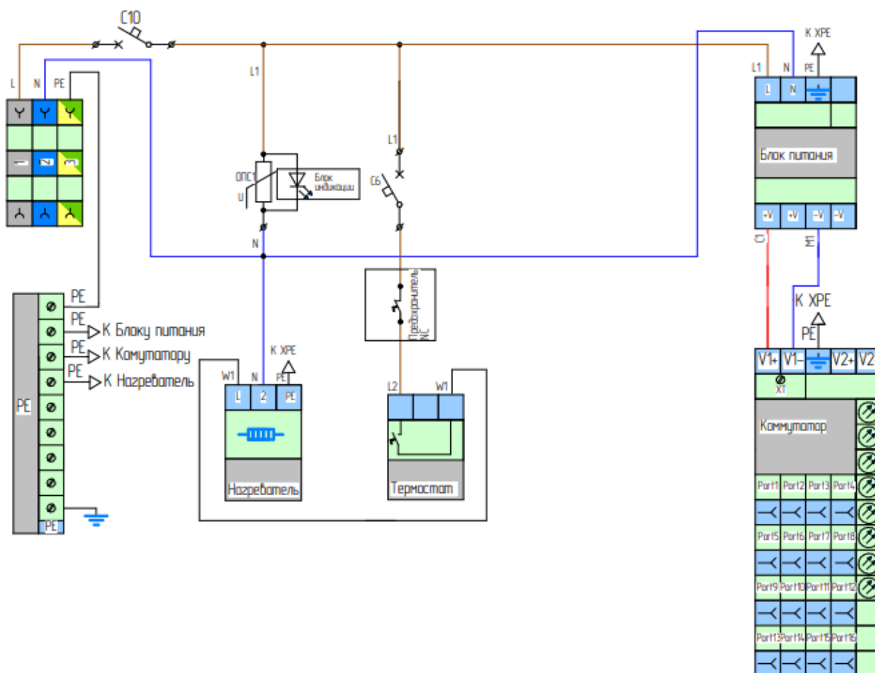
Рисунок 3. Электрическая схема Узла доступа 0168S1-PL
