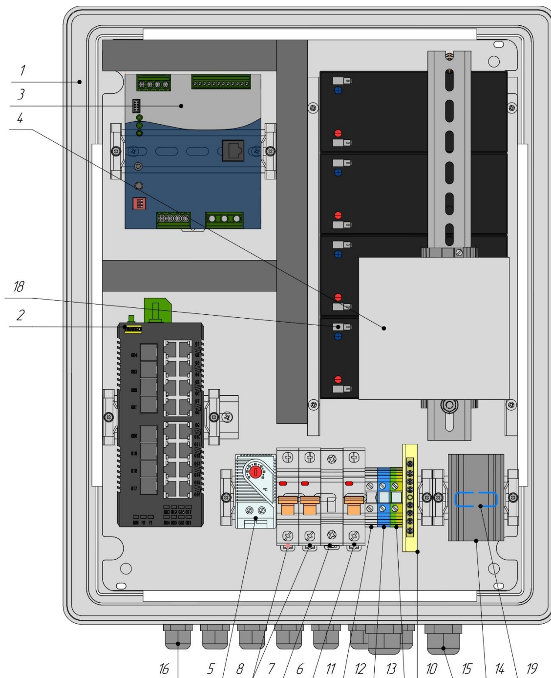
Рисунок 2. Схема расположения оборудования Узла доступа 0168S2-PL
