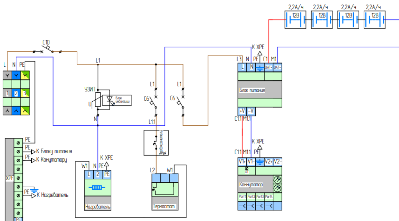
Рисунок 3. Электрическая схема Узла доступа 042S2-PL
