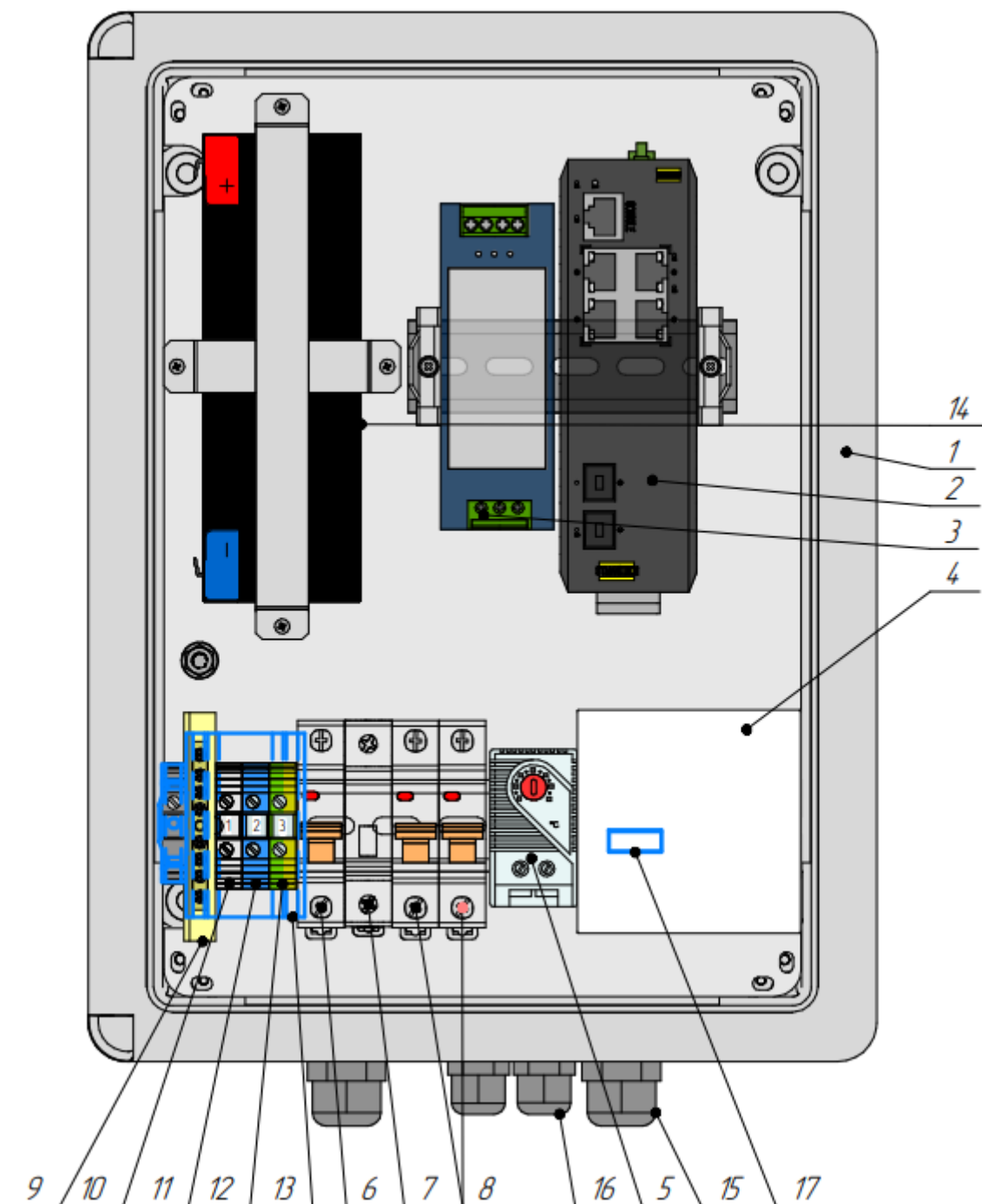
Рисунок 2. Схема расположения оборудования Узла доступа 042S2-PL
