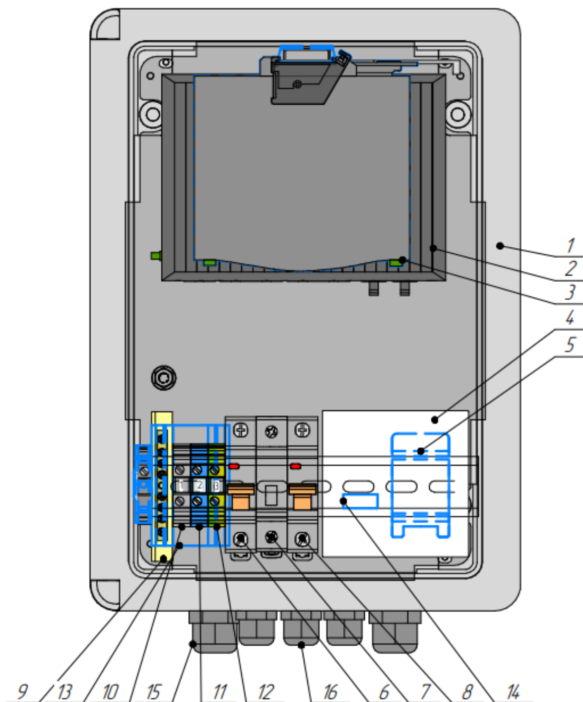
Рисунок 2. Схема расположения оборудования Узла доступа 082S1-PL
