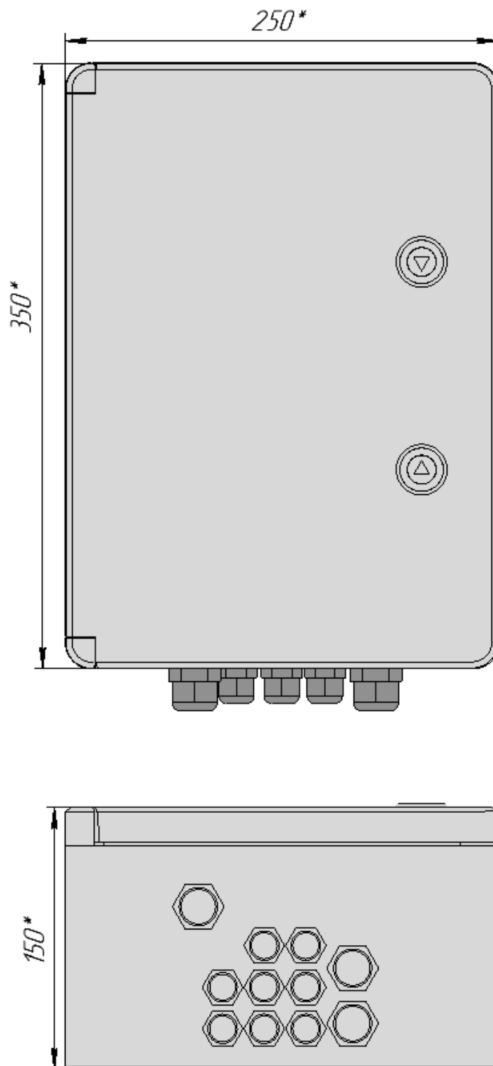
Рисунок 1 Внешний вид и габаритные размеры
