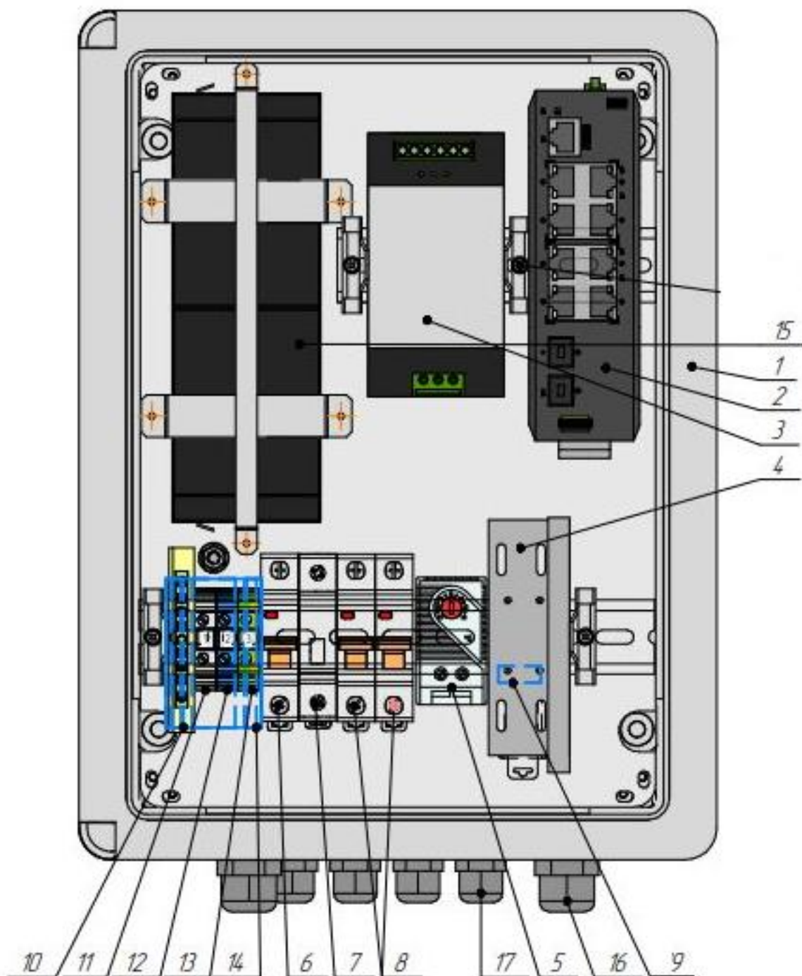
Рисунок 2. Схема расположения оборудования Узла доступа 082S2-PL
