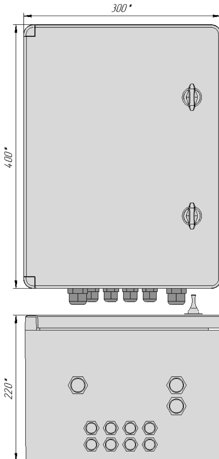
Рисунок .1 Внешний вид и габаритные размеры
