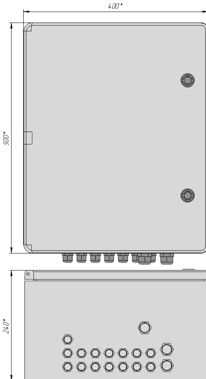
Рисунок 1. Внешний вид и габаритные размеры
