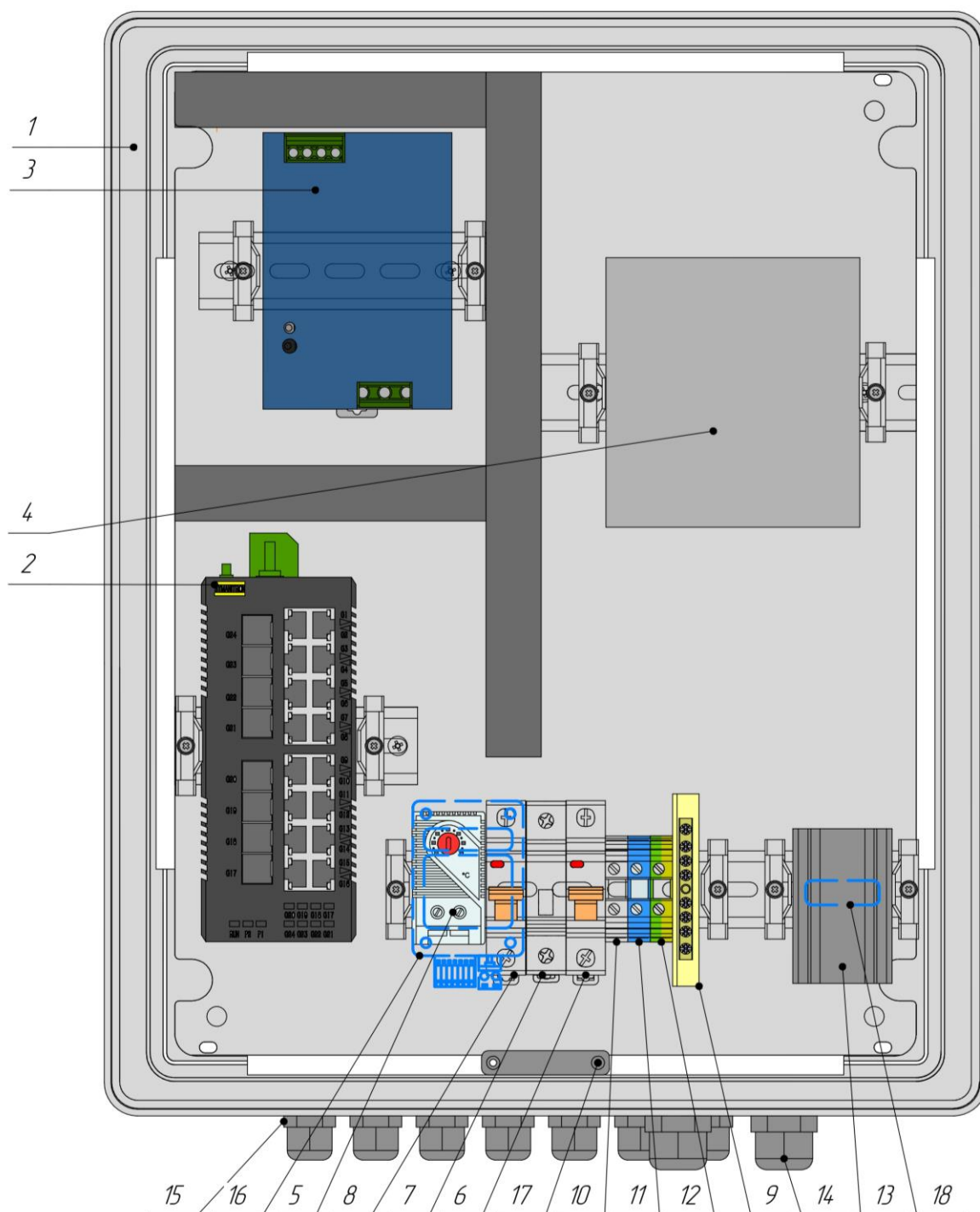
Рисунок 2. Схема расположения оборудования Узла доступа 1158S1-PL
