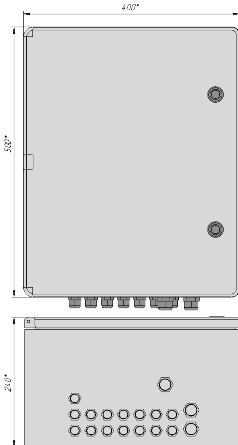
Рисунок 1. Внешний вид и габаритные размеры
