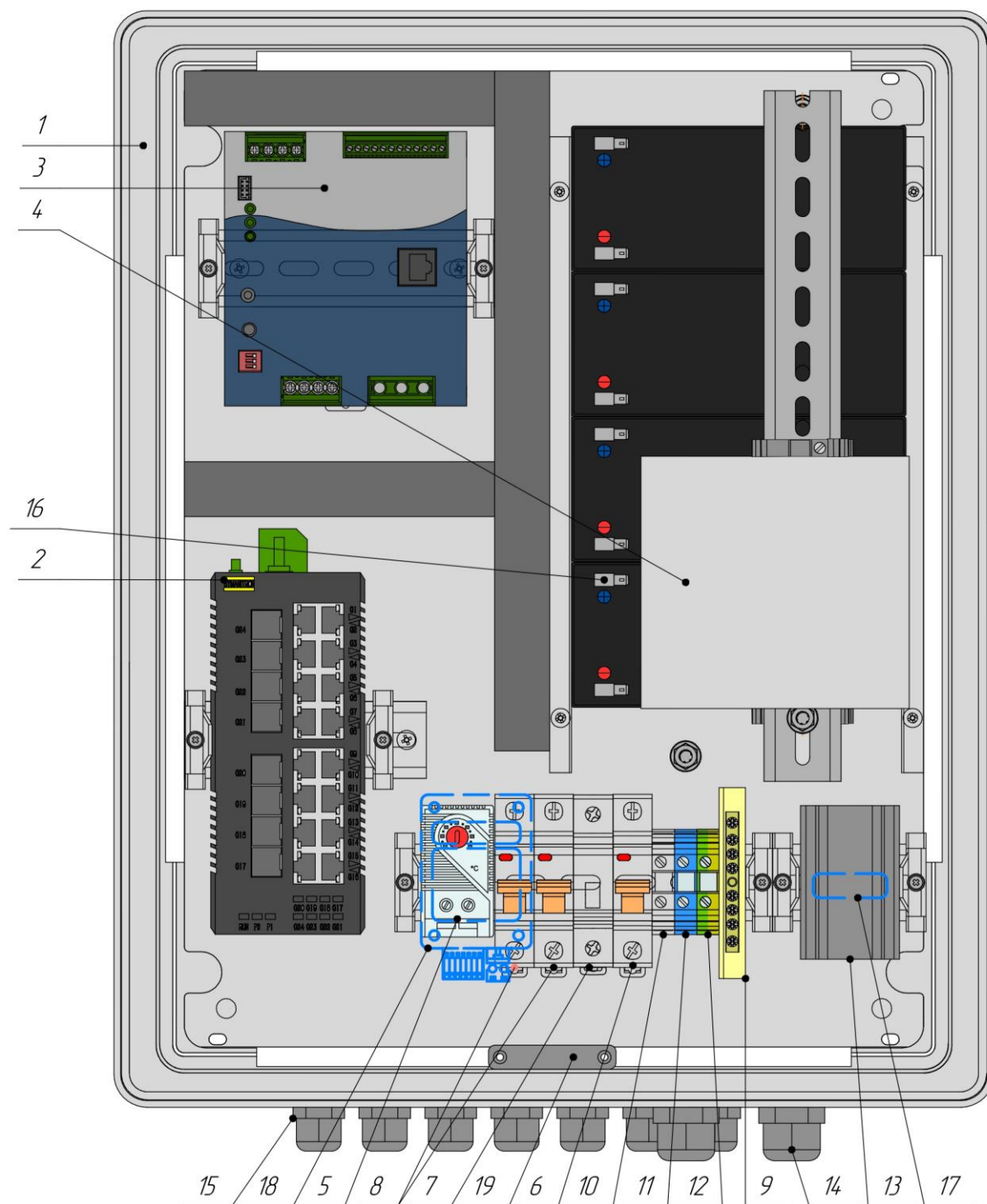
Рисунок 2. Схема расположения оборудования Узла доступа 1158S2-PL
