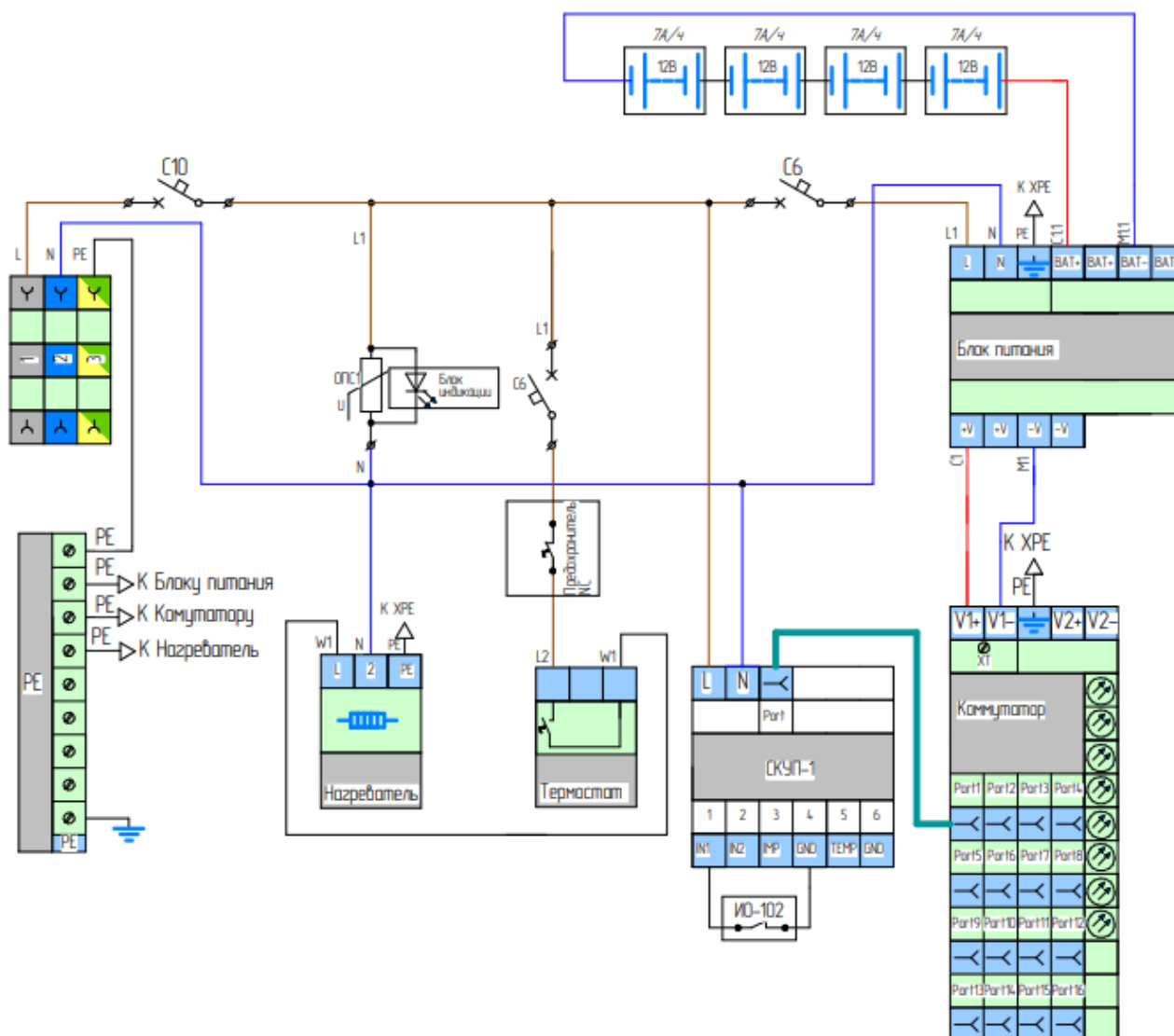
Рисунок 3. Электрическая схема Узла доступа 1158S2-PL
