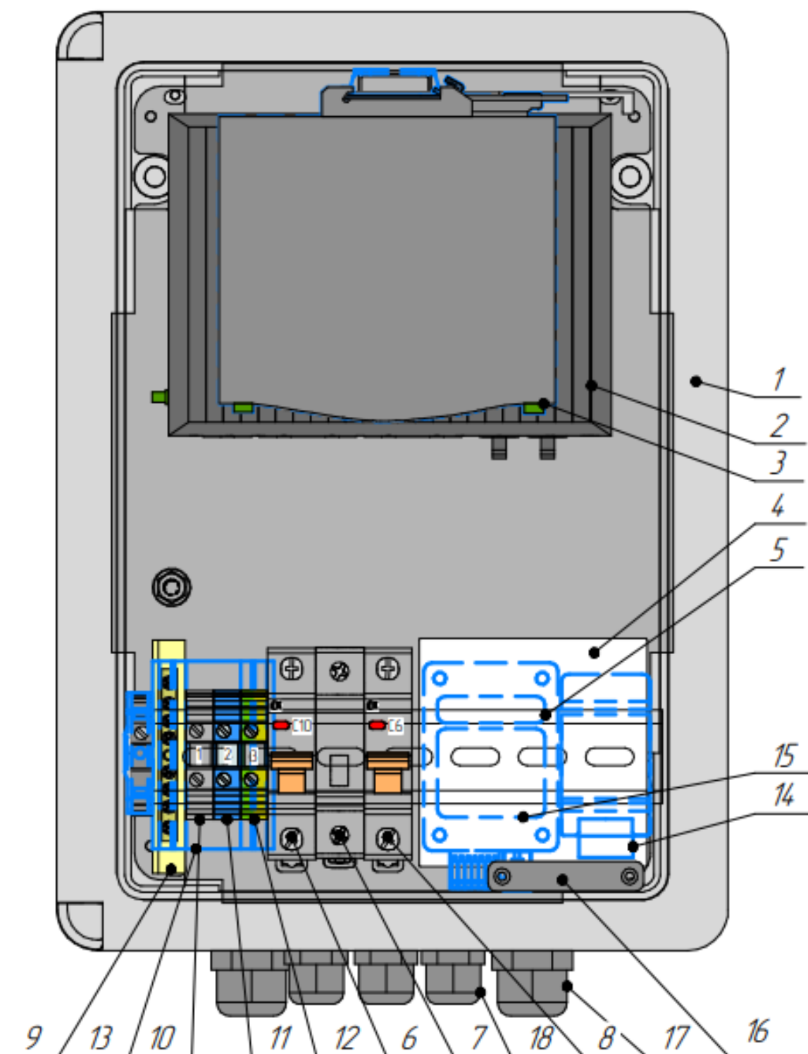
Рисунок 2. Схема расположения оборудования Узла доступа 172S1-PL
