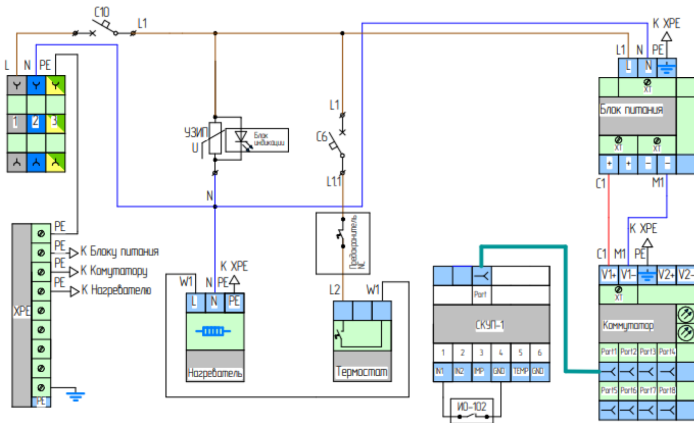
Рисунок 2. Электрическая схема Узла доступа 172SI-PL
