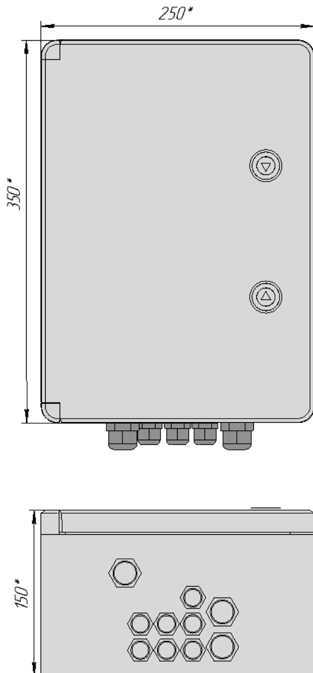
Рисунок 1. Внешний вид и габаритные размеры
