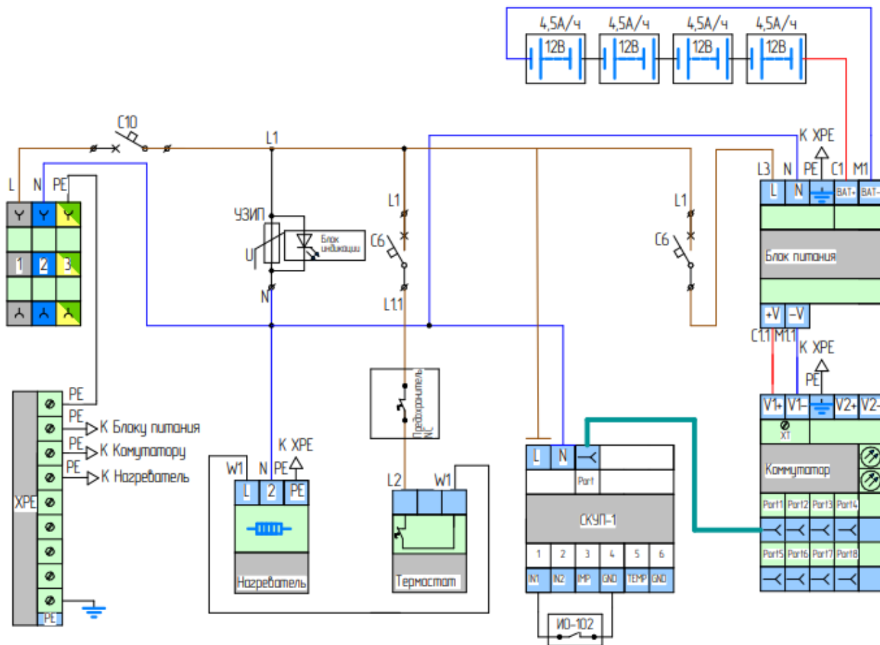
Рисунок 3. Электрическая схема Узла доступа 172S2-PL
