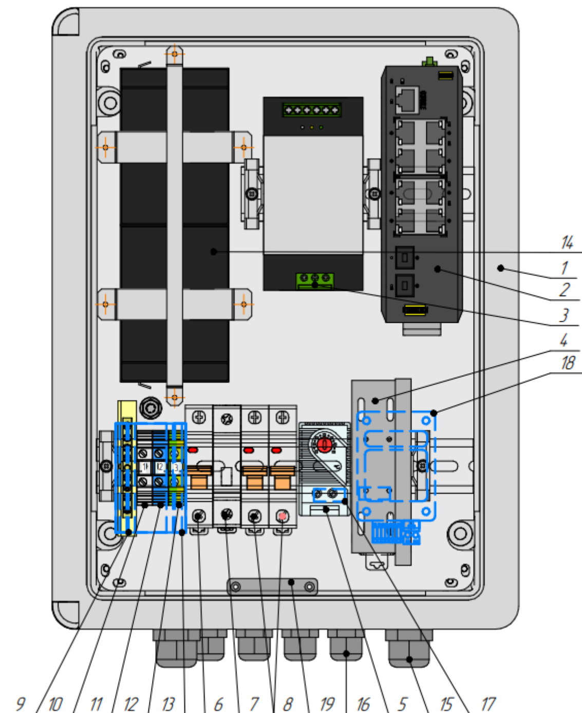
Рисунок 2. Схема расположения оборудования Узла доступа 172S2-PL
