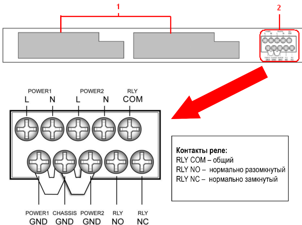
Рисунок 2 – Задняя панель
