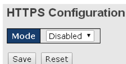
Рисунок 38 – Настройка режима HTTPS
