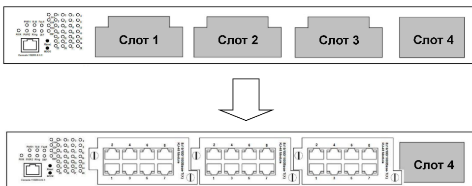
Рисунок 5 – Модули RJ-45
