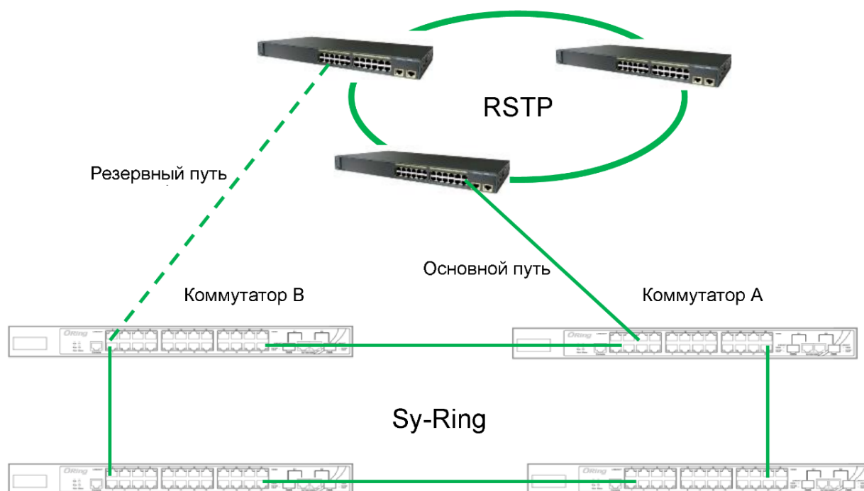
Рисунок 14 – Топология Dual Homing
