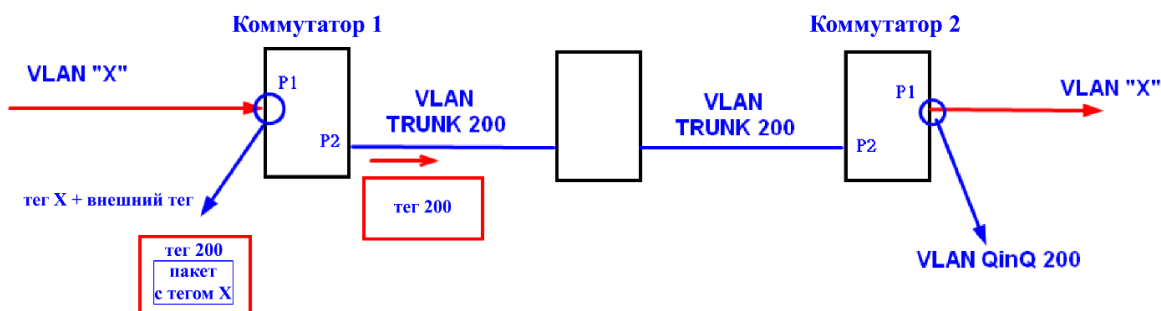
Рисунок 71 – QinQ
