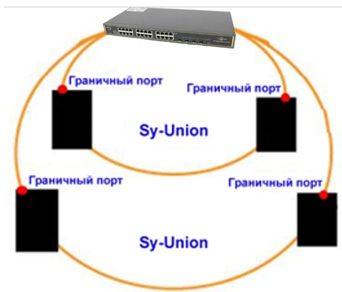
Рисунок 18 – Sy-Union
