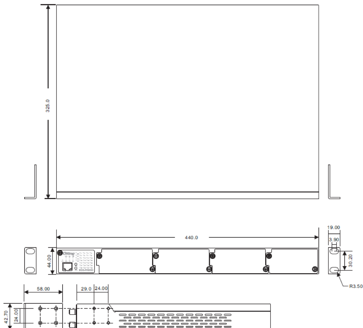
Рисунок 3 – Размеры установочного комплекта (единица измерения – мм)
