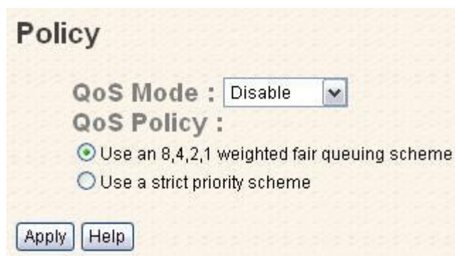
Рис. Интерфейс настройки политики
