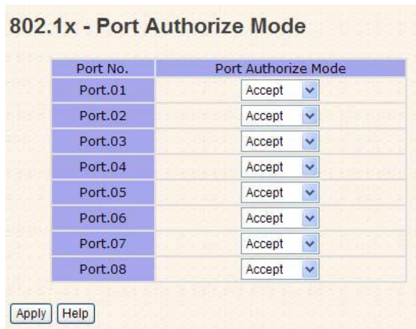
Рис. Интерфейс авторизованного порта 802.1x
