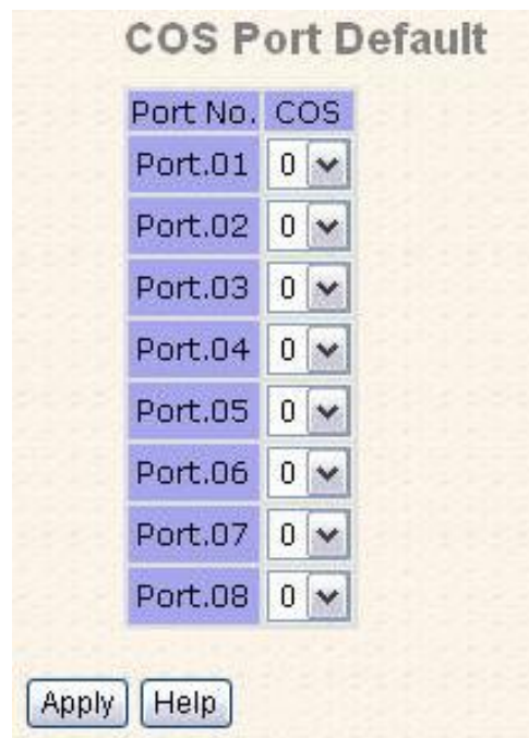
Рис. Интерфейс порта на основе приоритета
