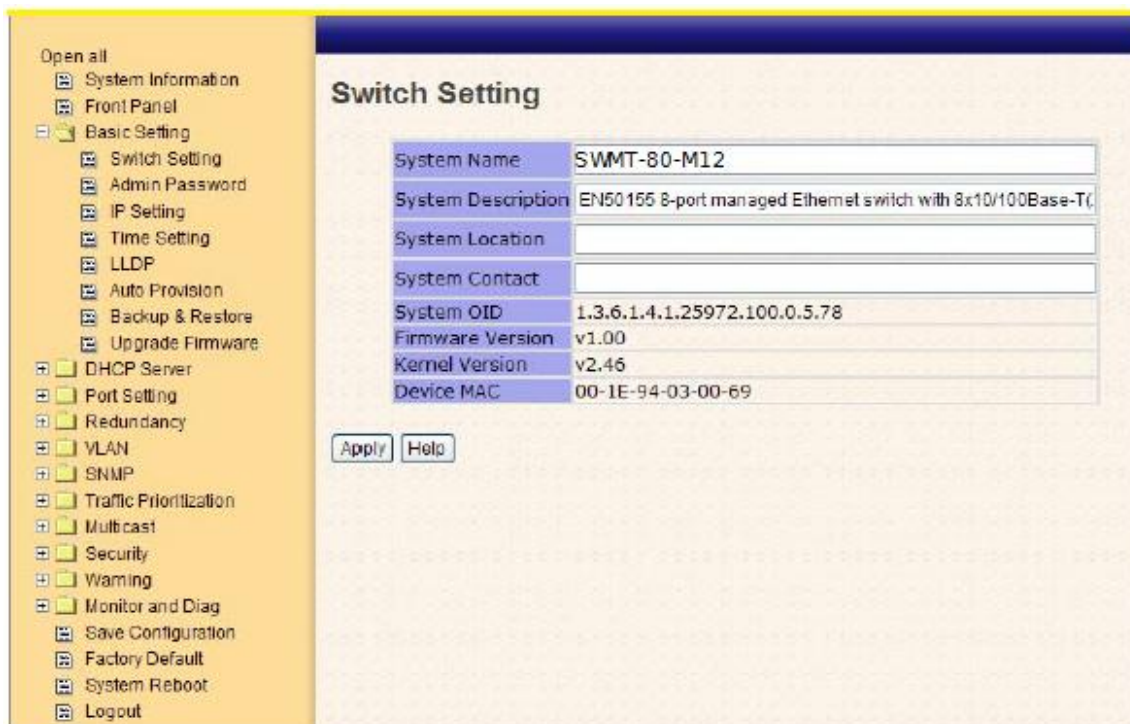
Рис. Настройки коммутатора
